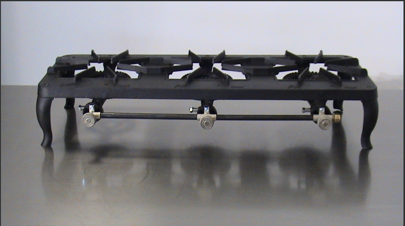
ΤΡΙΠΛΗ ΕΣΤΙΑ ΑΕΡΙΟΥ MOD. EUROPA
